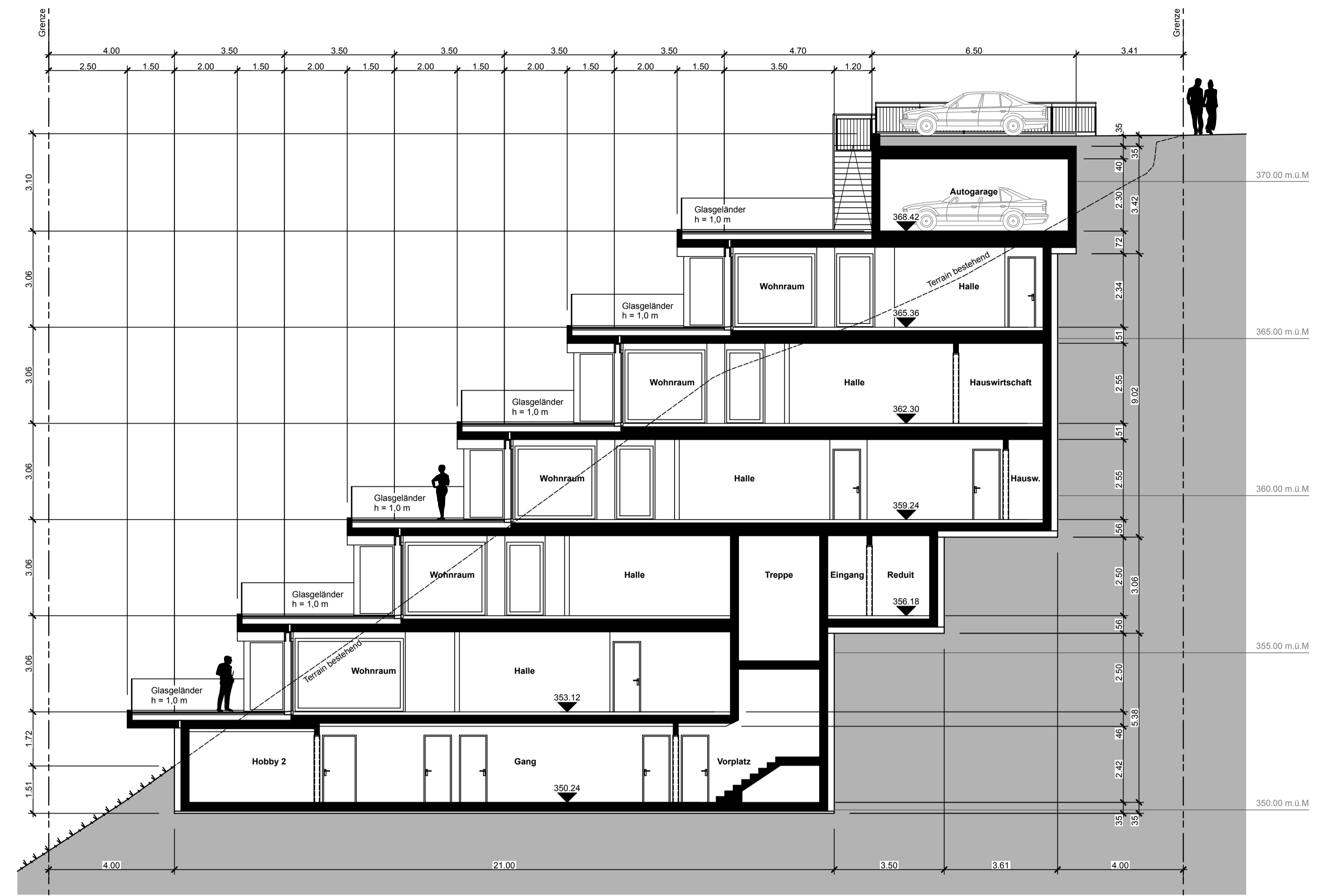
Schnitt S-A/A
