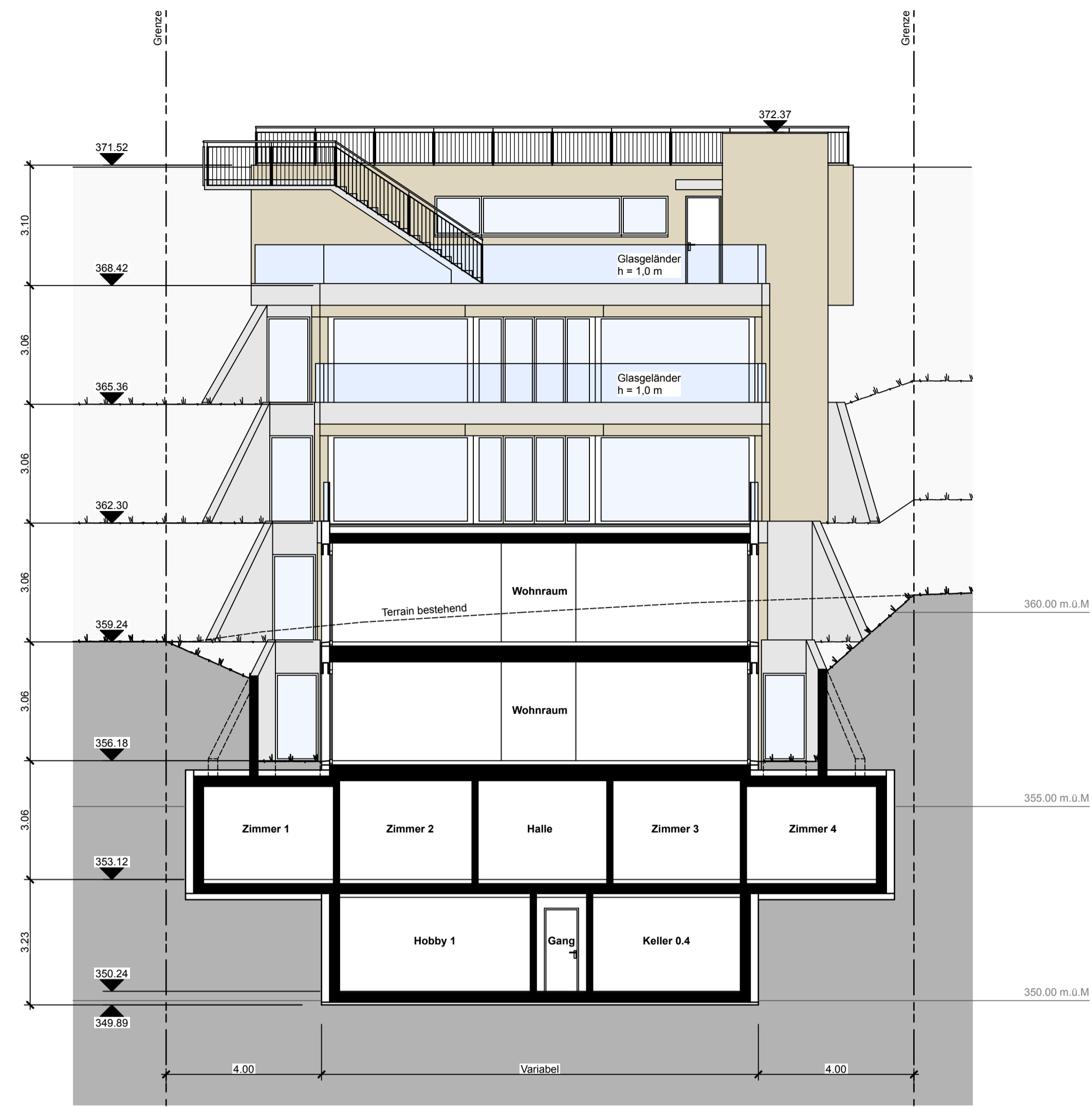
Schnitt S-B/B
